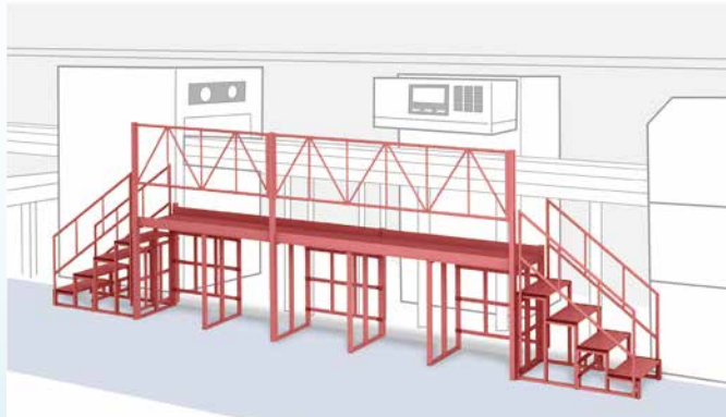
高所ライン作業台としての使用例
